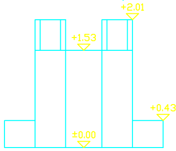
חתך 2 - 2
