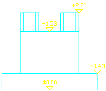
חזית צפונית
